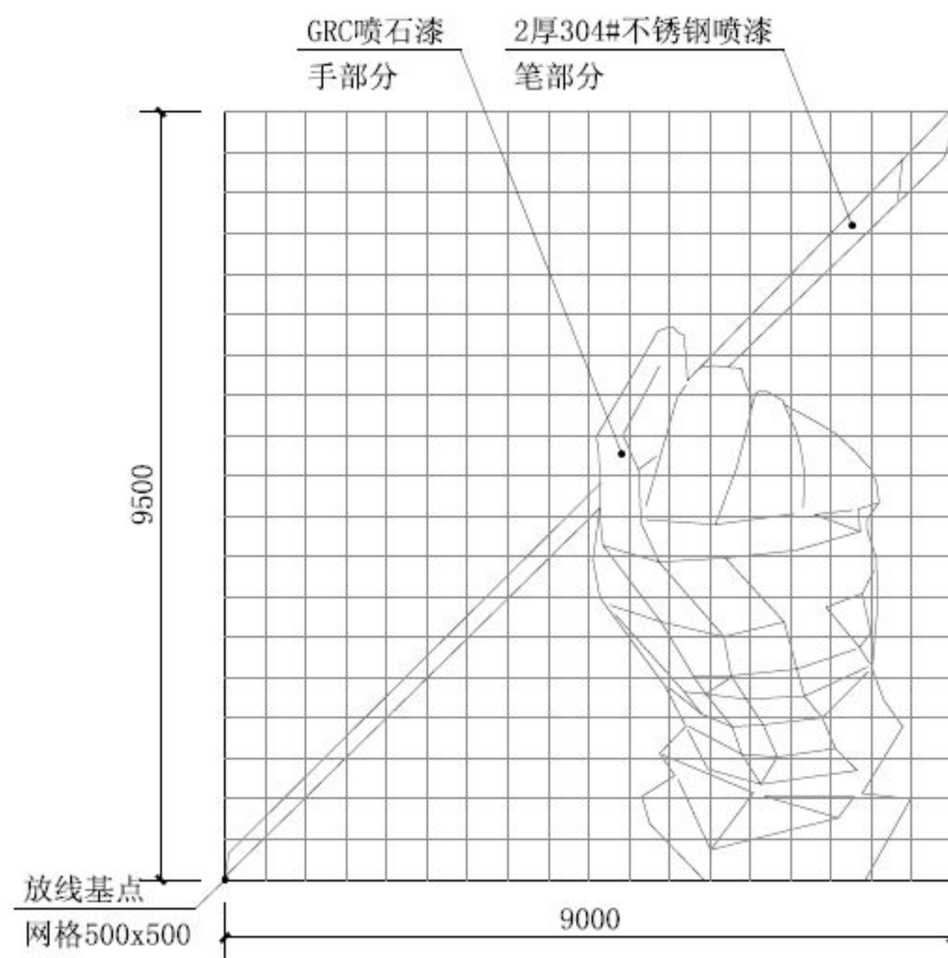
《达芬奇的手》网格放线图 1:100
