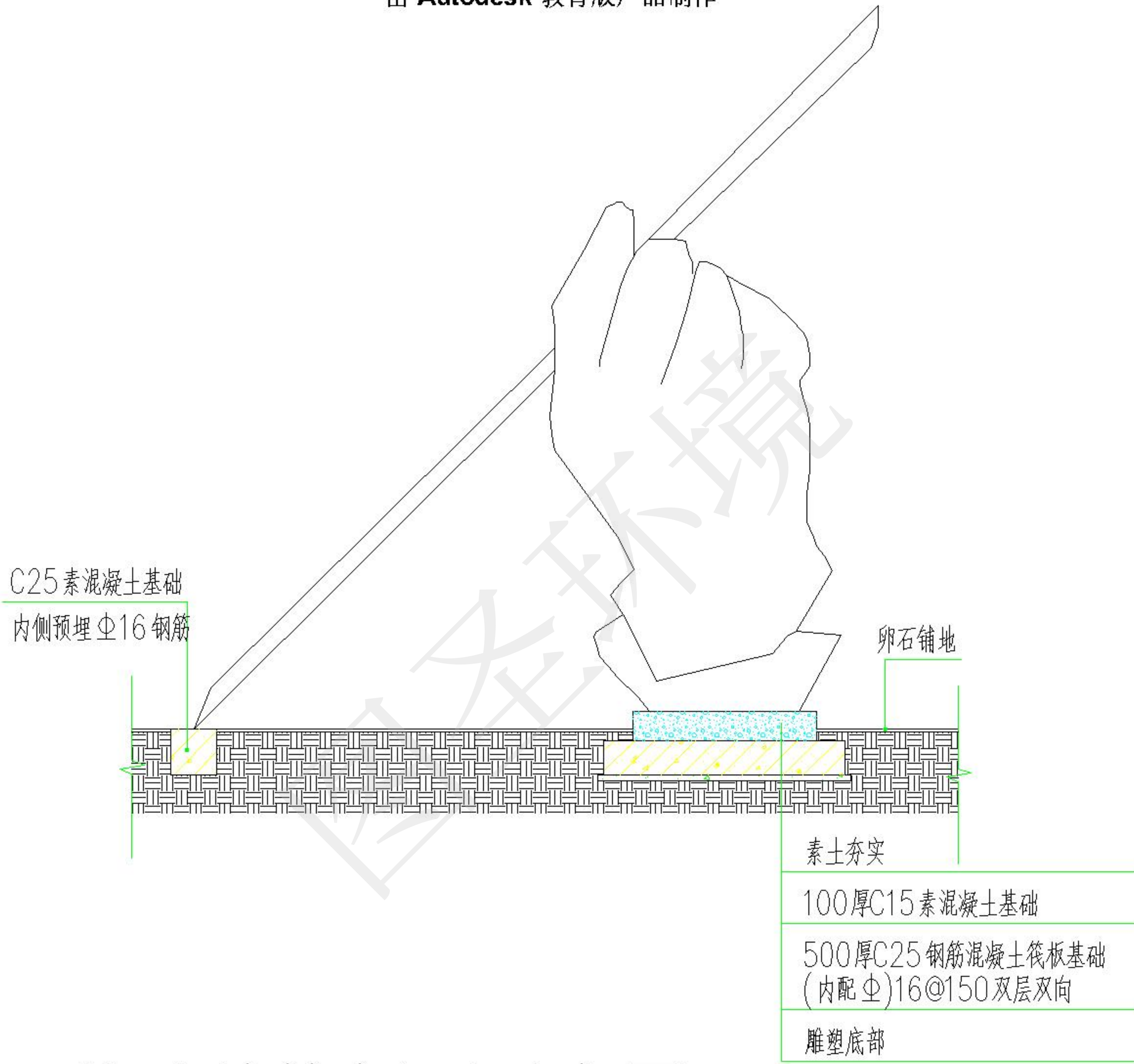
基础结构剖面示意图 1:100
