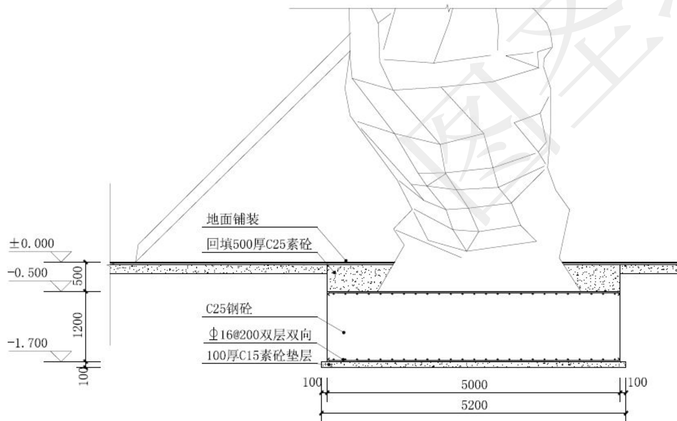
基础剖面图 1:60
