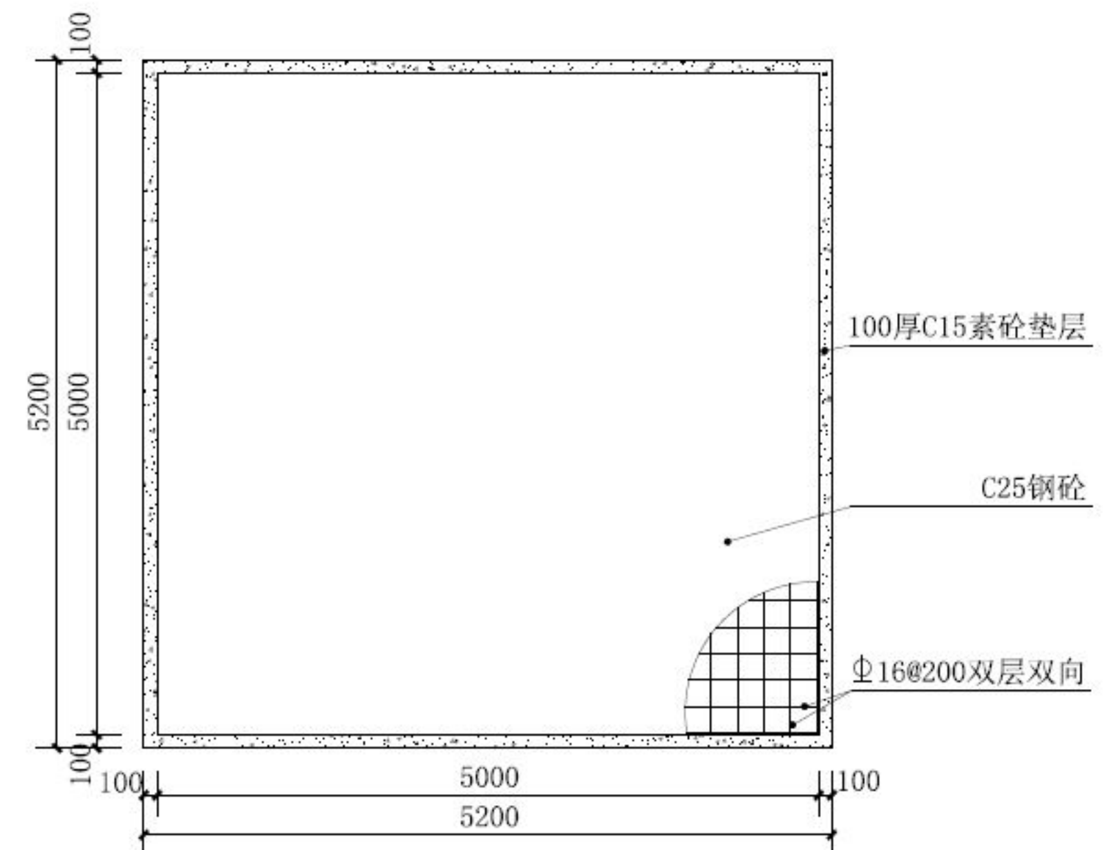
基础平面图 1:60
