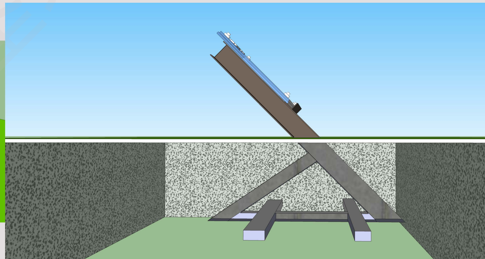
基础及预埋件设计
